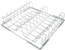
WB60D01 - Размер 600х500мм Кассета для тарелок на 24 шт. Ø 26 см WB60D02 - Размер 600х500мм Кассета для тарелок на 16 шт. Ø 32 см
