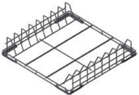
WB60T03 - Размер 600x500мм Кассета для 5 противней 600x400мм WB50T02 - Размер 500x500мм Кассета для 7 противней GN1/1 проф. 20мм
