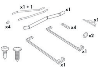
SVRPP625 Соединительный комплект для установки 2-х печей 6 уровней (600x400) и вытяжного зонта.
